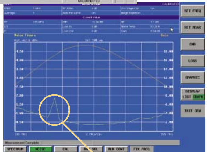
Rauschzahlmessung mit der Applikationsfirmware R&S®FS-K30
