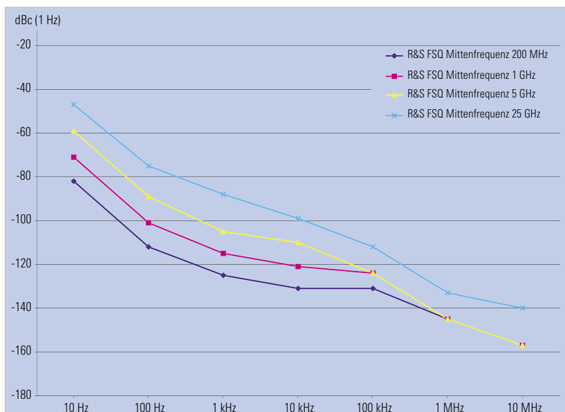
Phasenrauschen des R&S®FSQ bei verschiedenen Mittenfrequenzen
