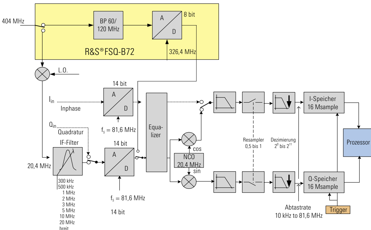
Prinzipieller Aufbau des Vektorsignalanalyseteils im R&S®FSQ
