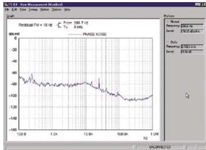
Phasenrauschmessung mit der Messsoftware R&S®FS-K4
