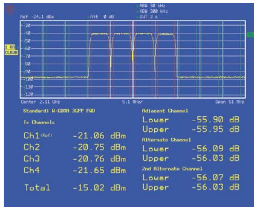
ACP Messung mit 4 Kanälen
