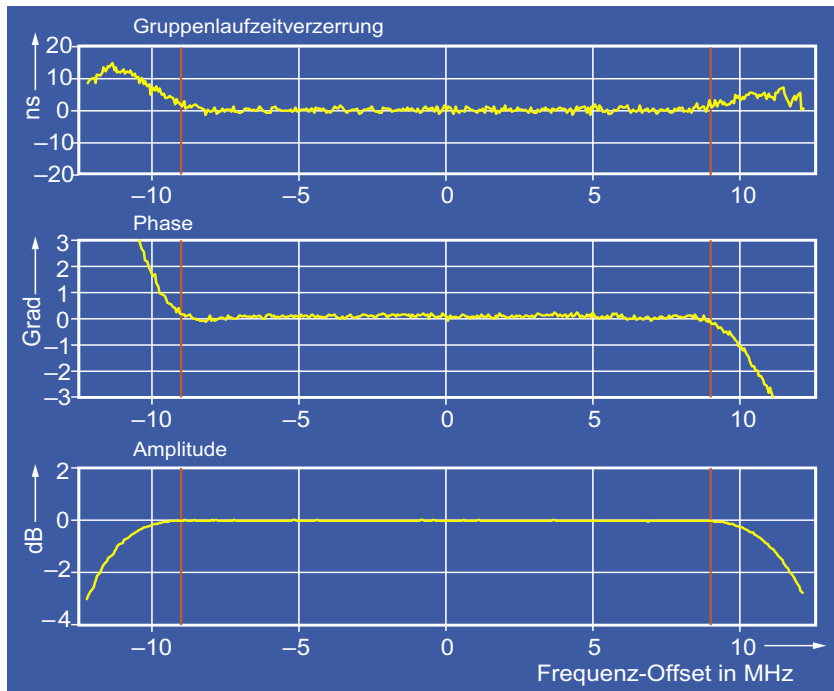
Frequenzgang und Gruppenlaufverzerrungen am Beispiel des 20-MHz-Auflösefilters
