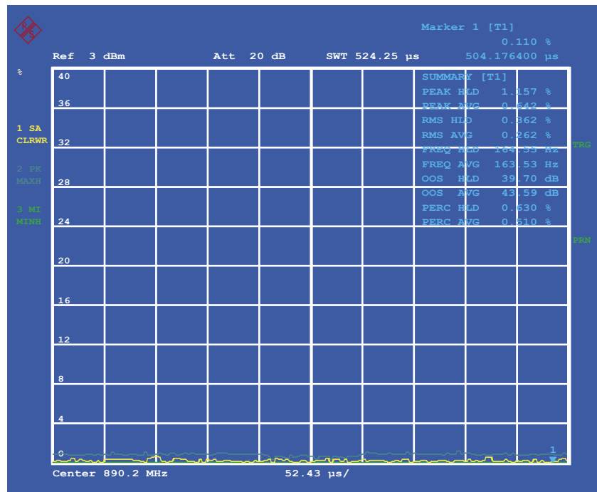
Messung von Modulation Accuracy an einem EDGE-Burst
