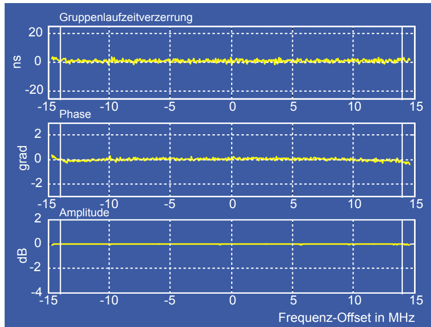
Frequenzgang und Gruppenlaufverzerrungen am Beispiel des 50-MHz-Auflösefilters
