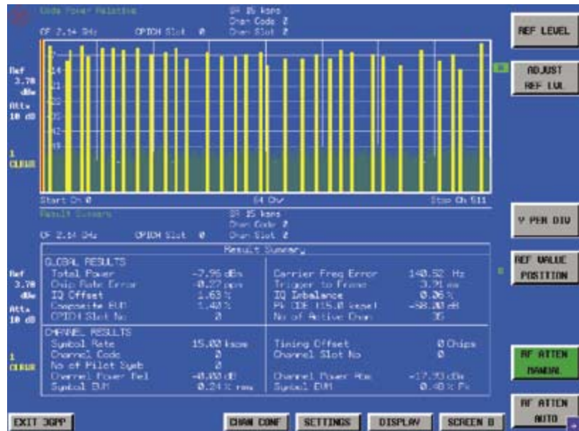
WCDMA-Code-Domain-Power-Messung mit R&S® FSQ und R&S® FS-K72
